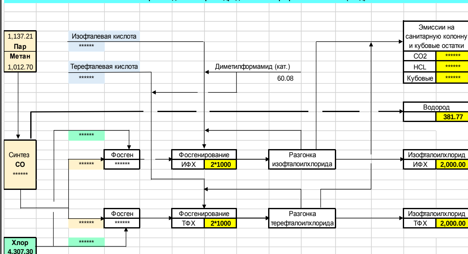
BFD схема производства хлорангидридов изо- и терефталевой кислот (т/год)
